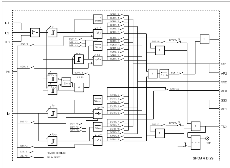
图 1. SPCJ 4D29 通用过流及接地保护继电器模块方框图
