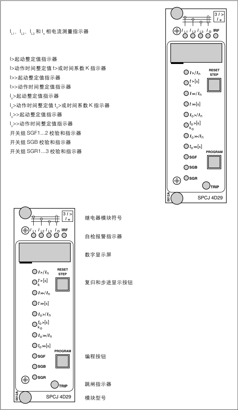
图2. SPCJ 4D29 通用过流及接地保护继电器模块的面板
