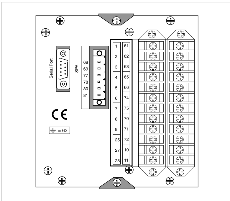
图 3. SPAJ 142C 继电器的端子排图（背视图）
