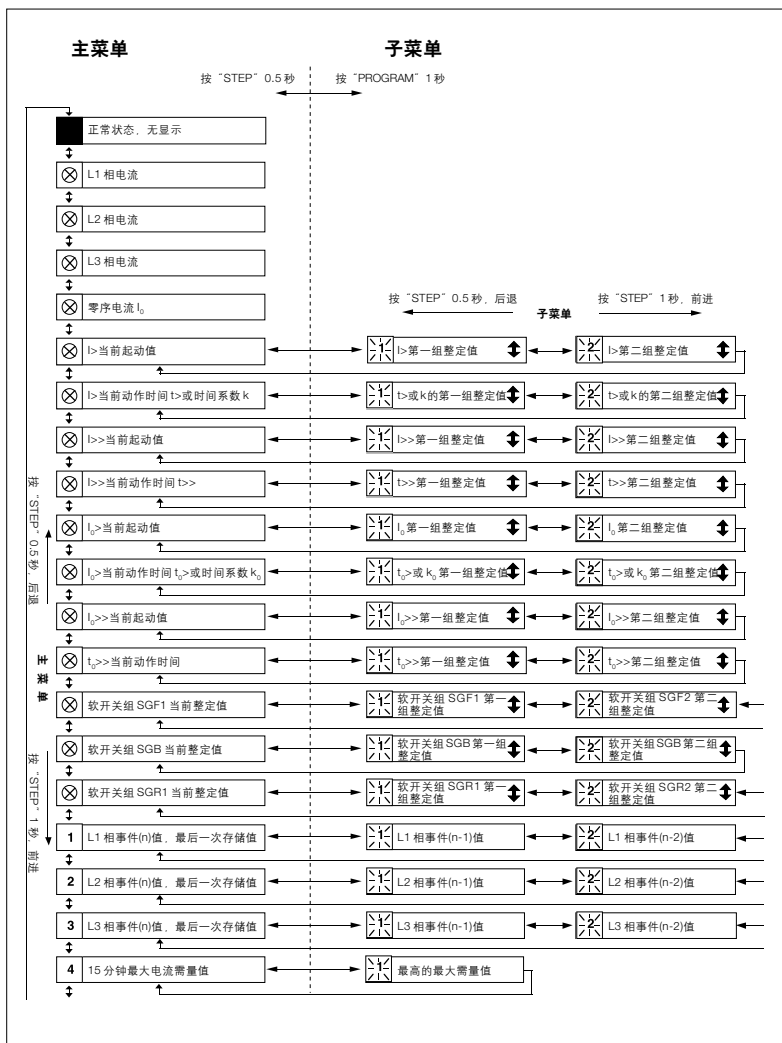
图 4. SPCJ 4D29 过流与接地故障模块部分整定用的主菜单和子菜单实例。当前整定值放在主菜单内，它们可按“STEP”按钮来显示。除了当前整定值外，主菜单还包含测量电流值，寄存器 1...9，0 和 A。所整定的第一组整定值与第二组整定值都放在子菜单中，要按编程按钮才能显示。
