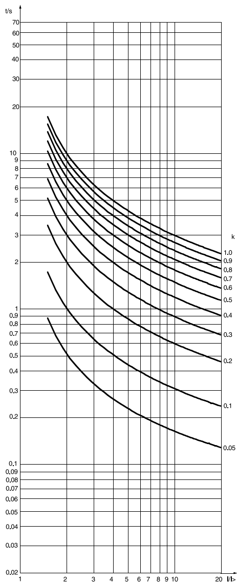
图 5. SPCJ 4D29 过流与接地故障单元的正常反时限特性曲线
