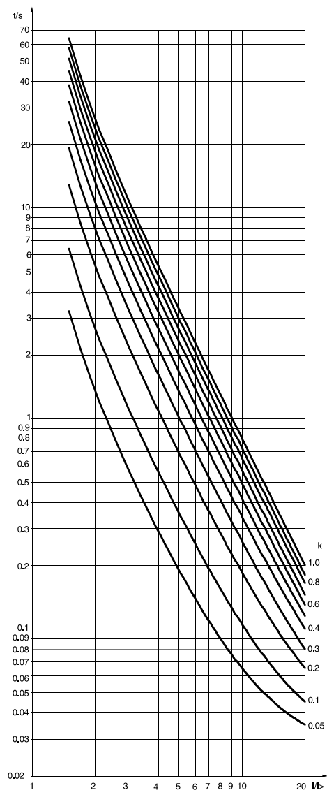
图 3. SPCJ 4D29 过流与零序电流单元的基反时限特性曲线
