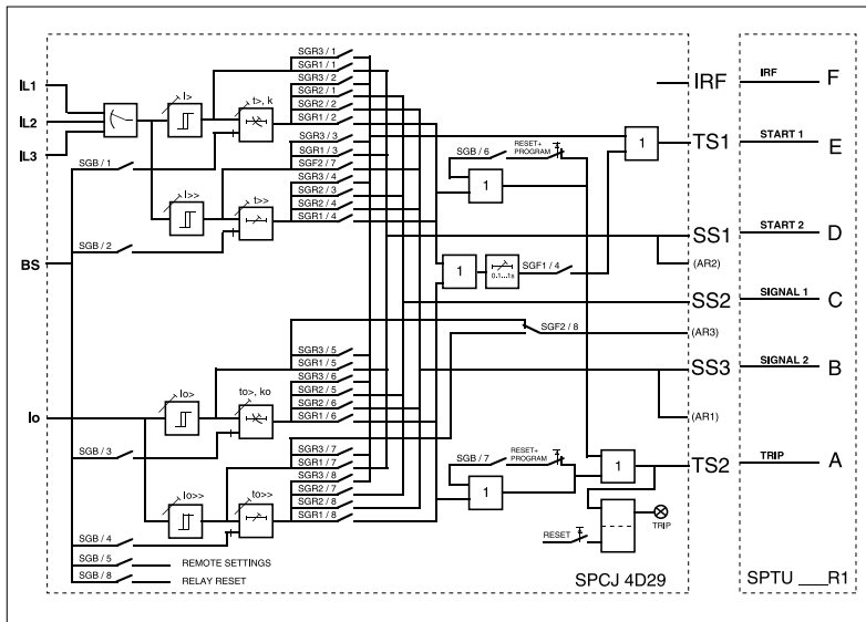
图 4. SPAJ 142C 过流及接地保护继电器模块之间的控制信号
