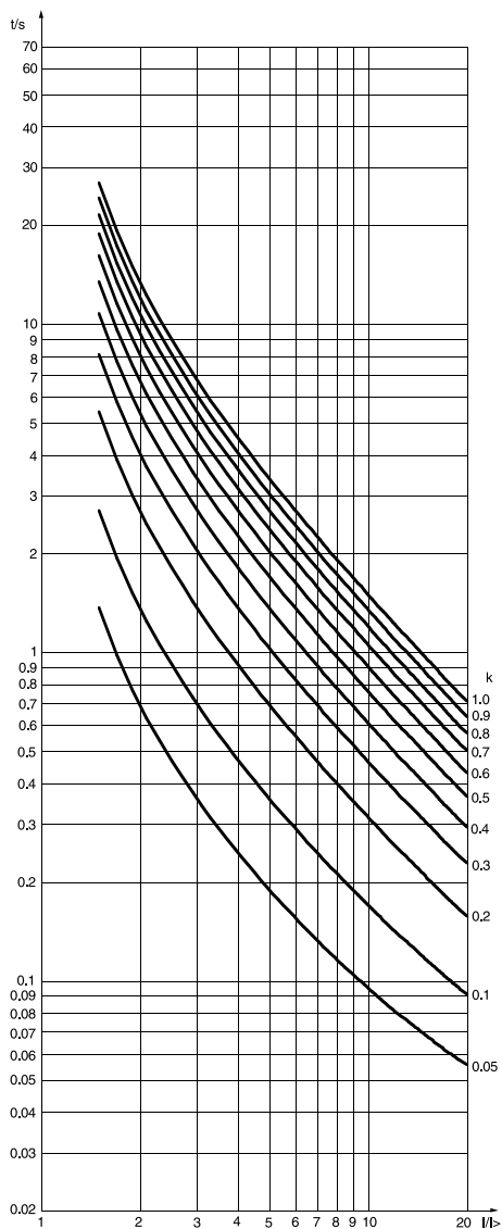
图 4. SPCJ 4D29 过流与接地故障单元的极反时限特性曲线
