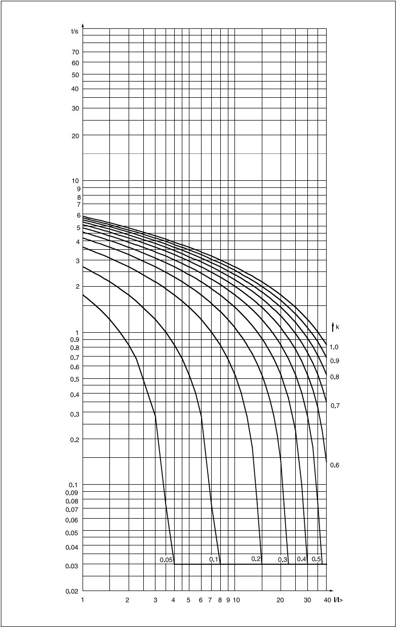
图 8. SPCJ 4D29 过流与接地故障单元的 RXIDG 型反时限特性曲线
