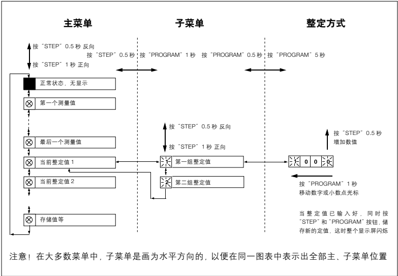
图3. 进入继电器模块主菜单和子菜单的基本原则
