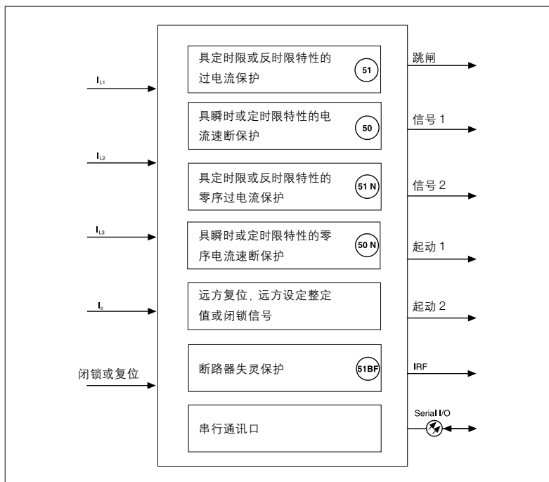
图 1. SPAJ 142C 过流与接地保护继电器的保护功能
