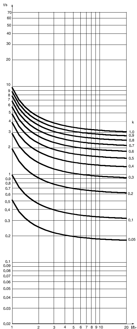
图 7. SPCJ 4D29 过流与接地故障单元的 RI 型反时限特性曲线
