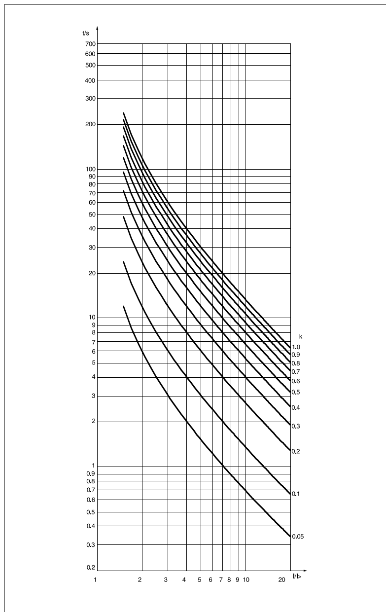
图 6. SPCJ 4D29 过流与接地故障单元的长反时限特性曲线
